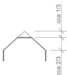
Obr. 3: Příklad přesahů střechy u štítové stěny na domech v Libníči - přesahy minimální
